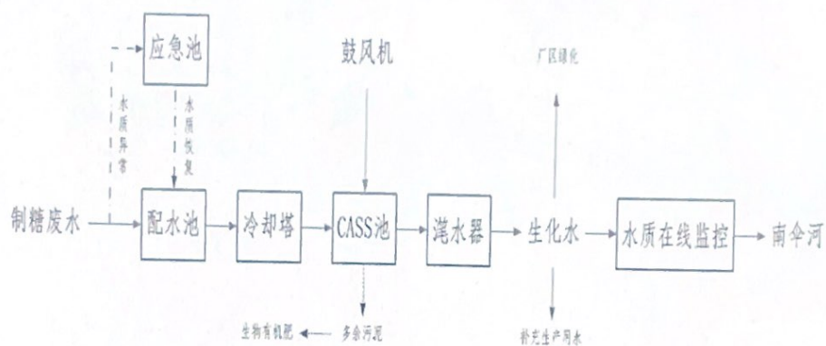
图 1 公司污水处理工艺流程图
