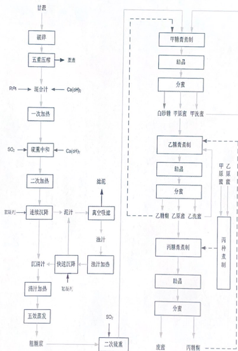
镇康南华南伞糖业有限公司白砂糖生产工艺流程图
