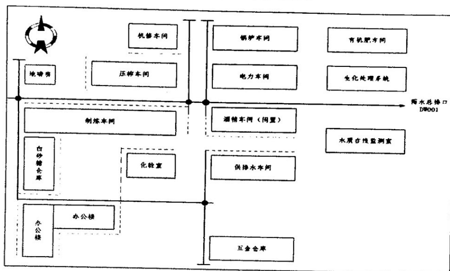
图 3 公司雨污分流图
