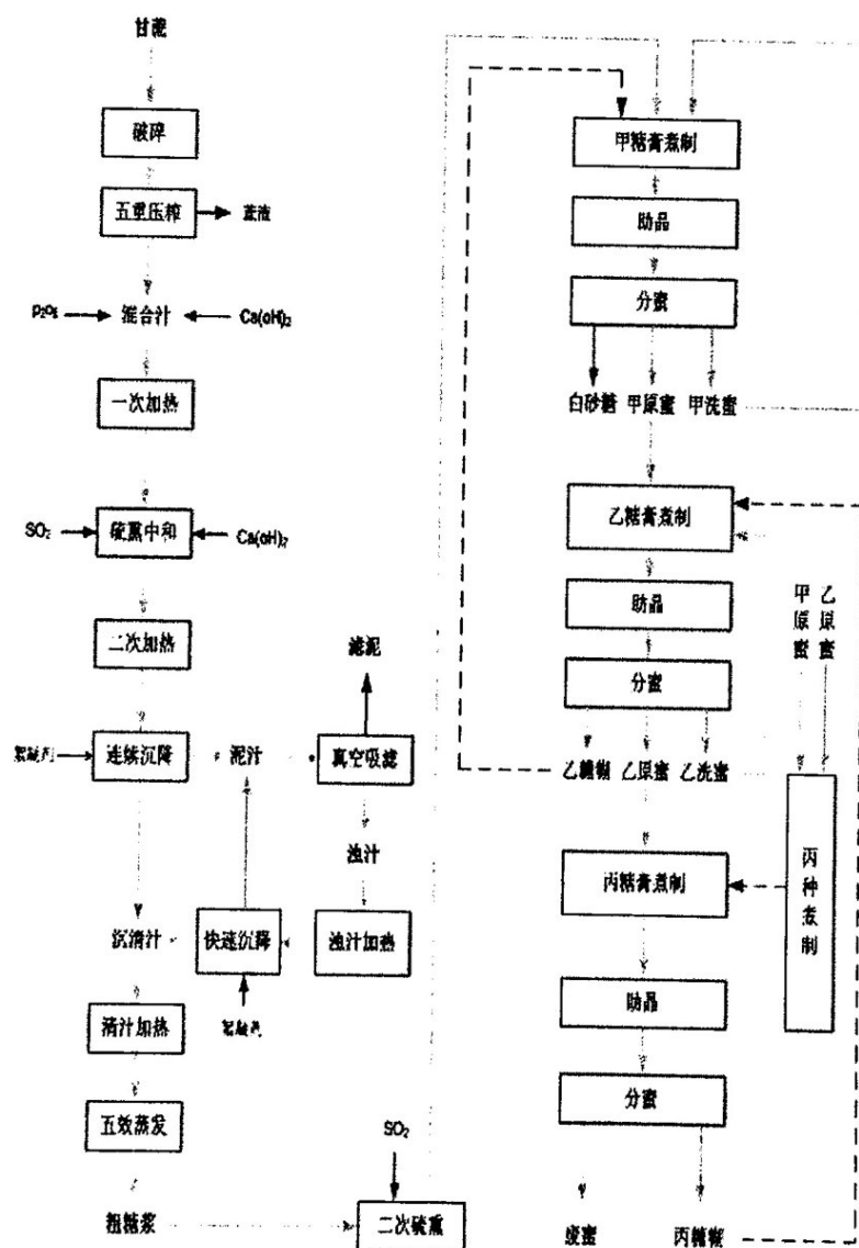
镇康南华南伞糖业有限公司白砂糖生产工艺流程图
