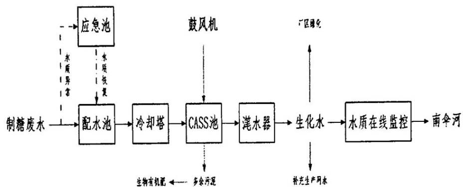
图1 公司污水处理工艺流程图
