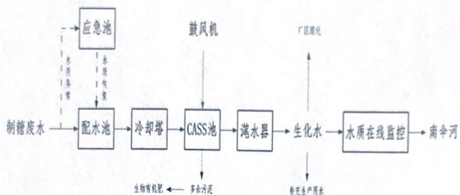
图1 公司污水治理工艺流程图
