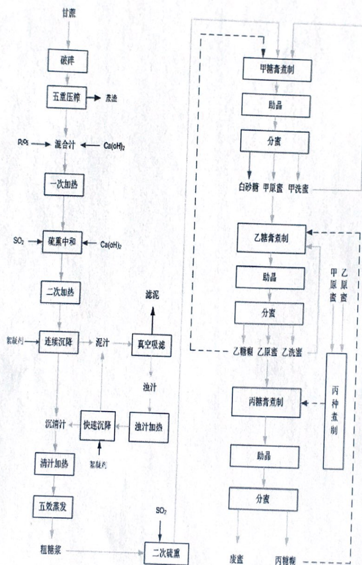
镇康南华南伞糖业有限公司白砂糖生产工艺流程图
