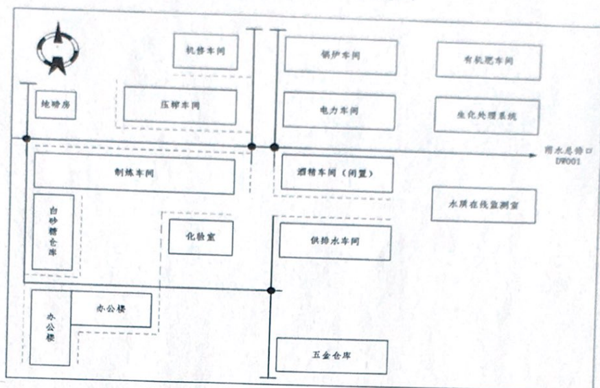
图3 公司雨污分流图
